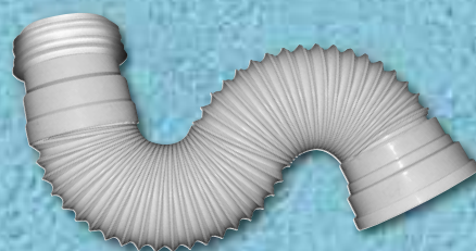
Racord WC extensibil cu manșon, armătură inox, D110, L=750 mm 167765
